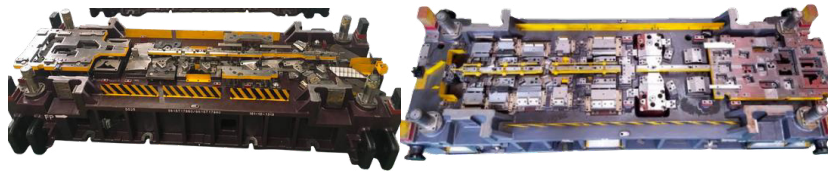
Troquel progresivo
