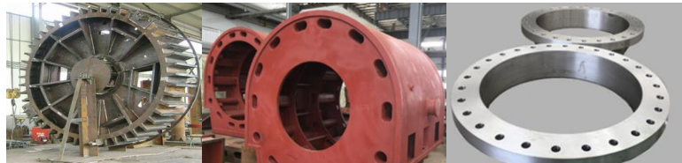
Estator del generador
